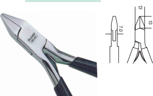
Бокорезы (110 мм)
