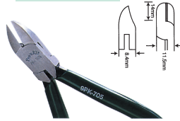
Бокорезы (125 мм)
