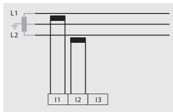
Рис. Показатели входа для измерения тока I3 приравниваются к нулю и не рассчитываются.
